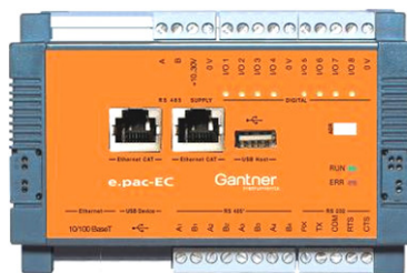
e.pac EC
